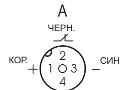
Цоколевка соединителя CS S20-5- -C
