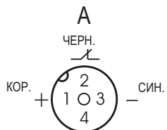
Цоколевка соединителя CS S20-5- -C
